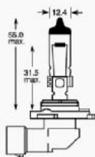
H12 Pz20d
