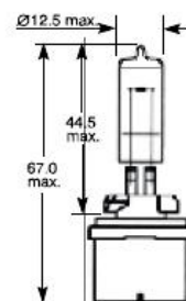
PG13
