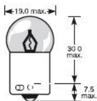
BAU15s
