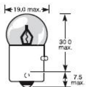
RR5W BAW15s
